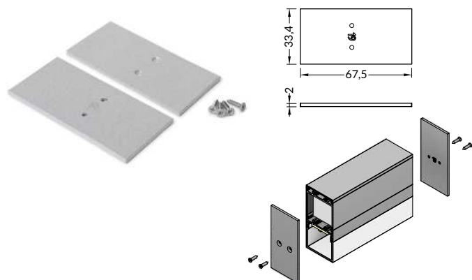
Endkappe VARIO30-19-E9 aus Metall / VARIO30-19-E9 metal ending
