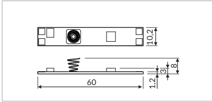
LED Berührungsschalter INSIDE dimmbar LED switch INSIDE touch dimmable 12-24 V; 60-100 W
