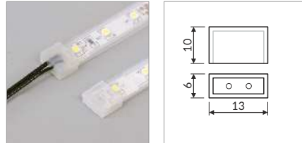
Endkappe für die Silikonhülle für LED Streifen mit 8 mm ending for silicone housing for 8 mm LED strip
