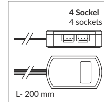
LED RGB integrierter Verteiler RGB LED distribution box 4x0,5 200 mm 4xMIKRO4 Sockel / 4xMIKRO4 socket
