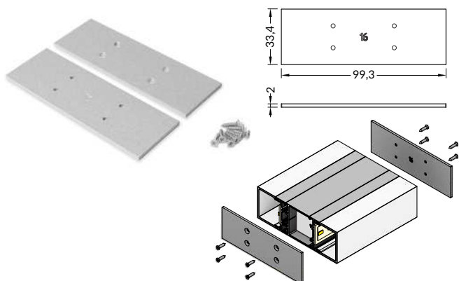
Endkappe VARIO30-16-E9 aus Metall / VARIO30-16-E9 metal ending
