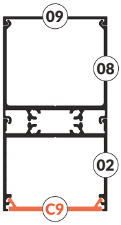
Variante 27 - Hängeversion 09-08-02-C9 variant 27 - pendant 09-08-02-C9
