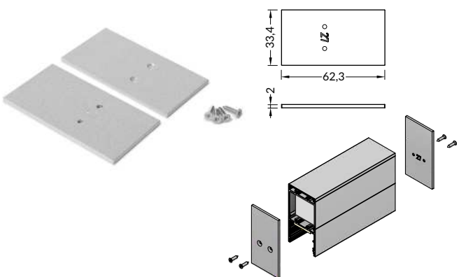
Endkappe VARIO30-27 aus Metall / VARIO30-27 metal ending
