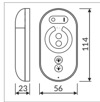
LED Fernbedienung warmweiß-kaltweiß LED remote controller warm-cold
