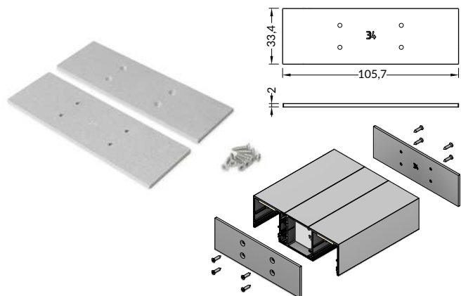
Endkappe VARIO30-34 aus Metall / VARIO30-34 metal ending
