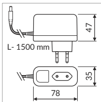
18 W 12 V / 100-240 V Netzteil für LED mit Stecker / AC adapter
