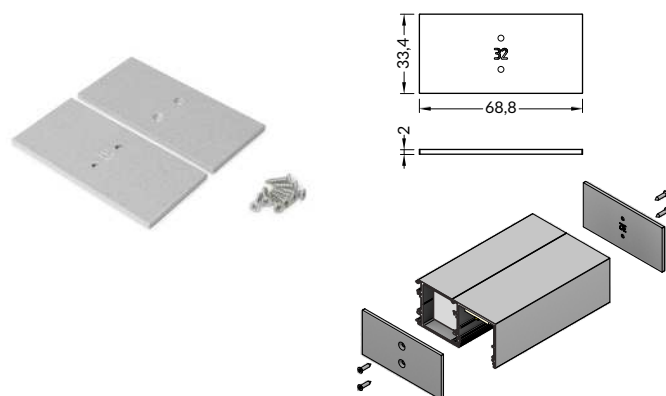
Endkappe VARIO30-32 aus Metall / VARIO30-32 metal ending
