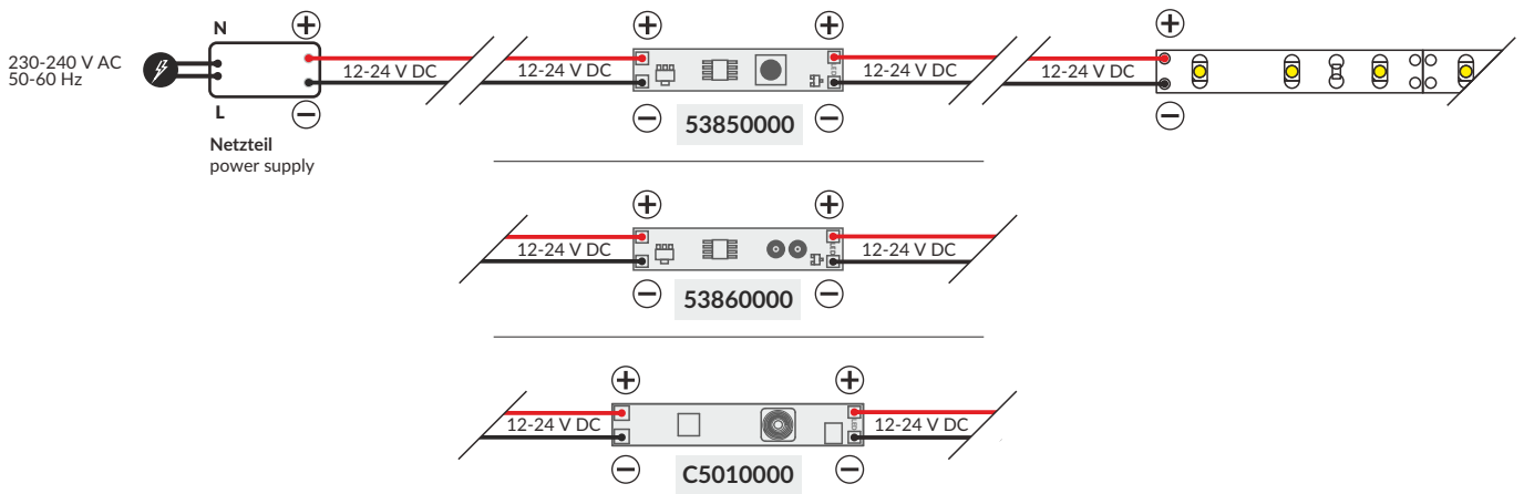
LED Berührungsschalter INSIDE dimmbar LED switch INSIDE touch dimmable 12-24 V; 60-100 W
