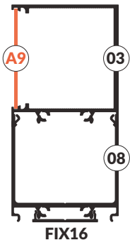
Variante 32 - seitliche Wandversion FIX16-08-03-A9 variant 32 - wall side FIX16-08-03-A9
