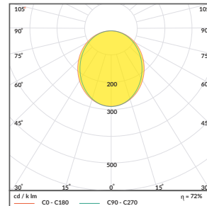
Der Vergleich von Lichtverteilungskurven bei der Anwendung von unterschiedlichen C10 Abdeckungen Comparison of variations in the light curves measured on different C10 covers
