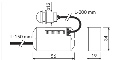
Bewegungssensor YCB1050 movement sensor YCB1050 230 V; 800 W
