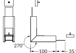
270 deg bent / deg bent
